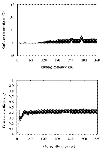
圖 8 CrO 2 在 80N 及 200mm/s 條件下之動態摩擦係數與表面磁場的響應
