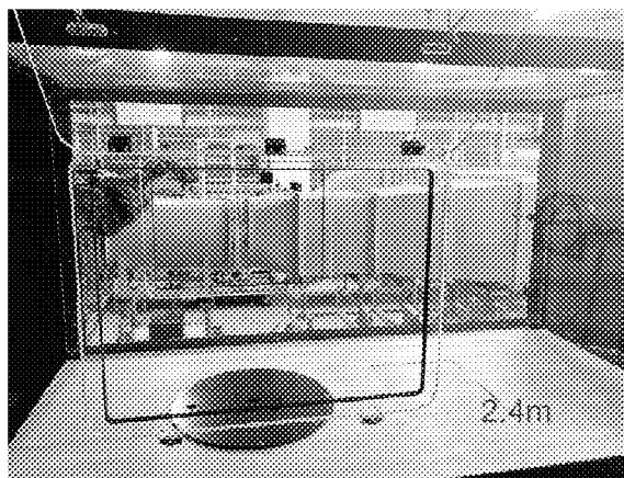
試驗段：管內總長2.4m · 管內高1.2m · 管內寬1.2m
