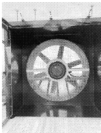
試驗段：管內總長2.4m · 管內高1.2m · 管內寬1.2m
